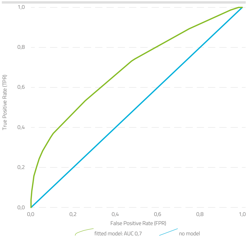
Abbildung 2: Modellgütevalidierung in Form einer ROC-Analyse
